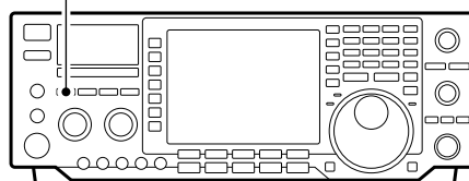
[TUNER] 2 Sek. gedrückt halten
