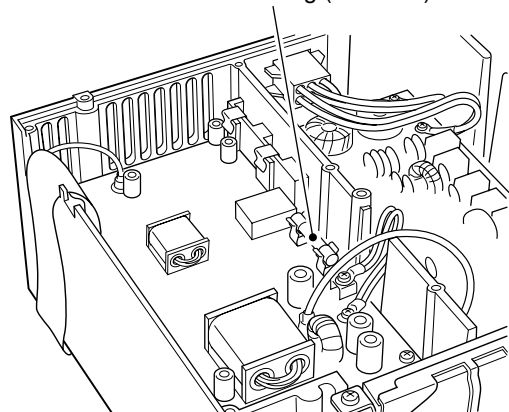
Platinen-Sicherung (FGB 5 A)
